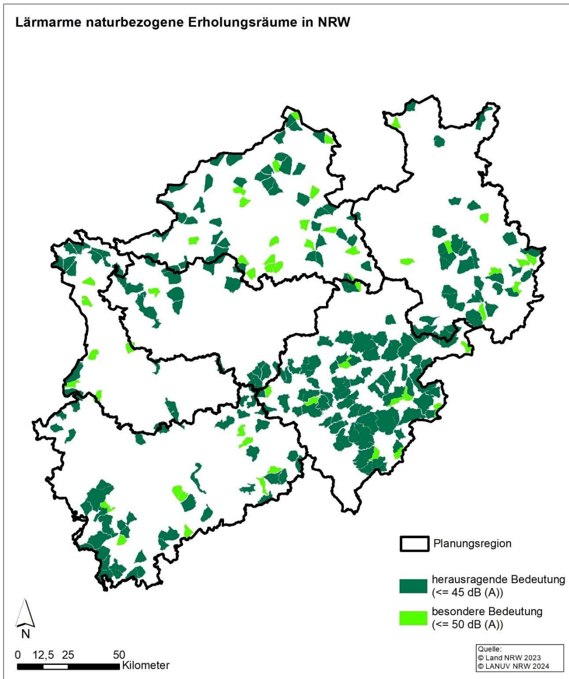
Abb. 13 Lärmarmer naturbezogene Erholungsräume in Nordrhein-Westfalen (LAND NRW 2023, LANUV 2024)
